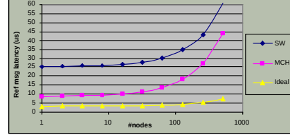
Fig. 2. 256B msg latency vs. cluster size
